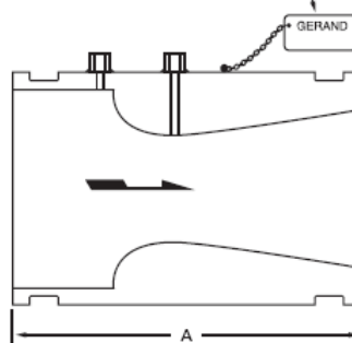
Model Venturi, butt weld, grooved ends/Anschweißenden, geriefte Enden/Raccordements rainurés ou soudés
